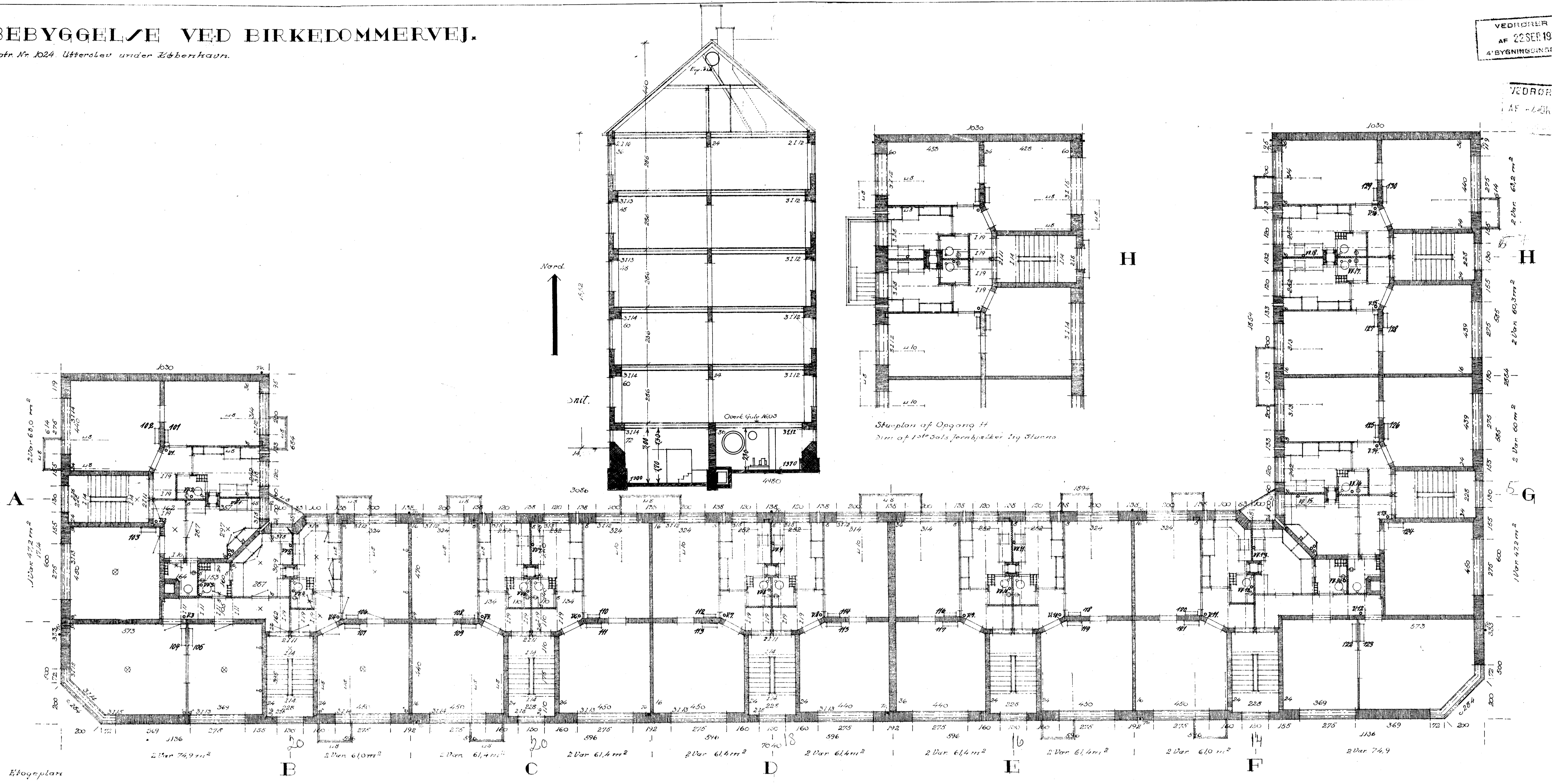
Etagetplan
