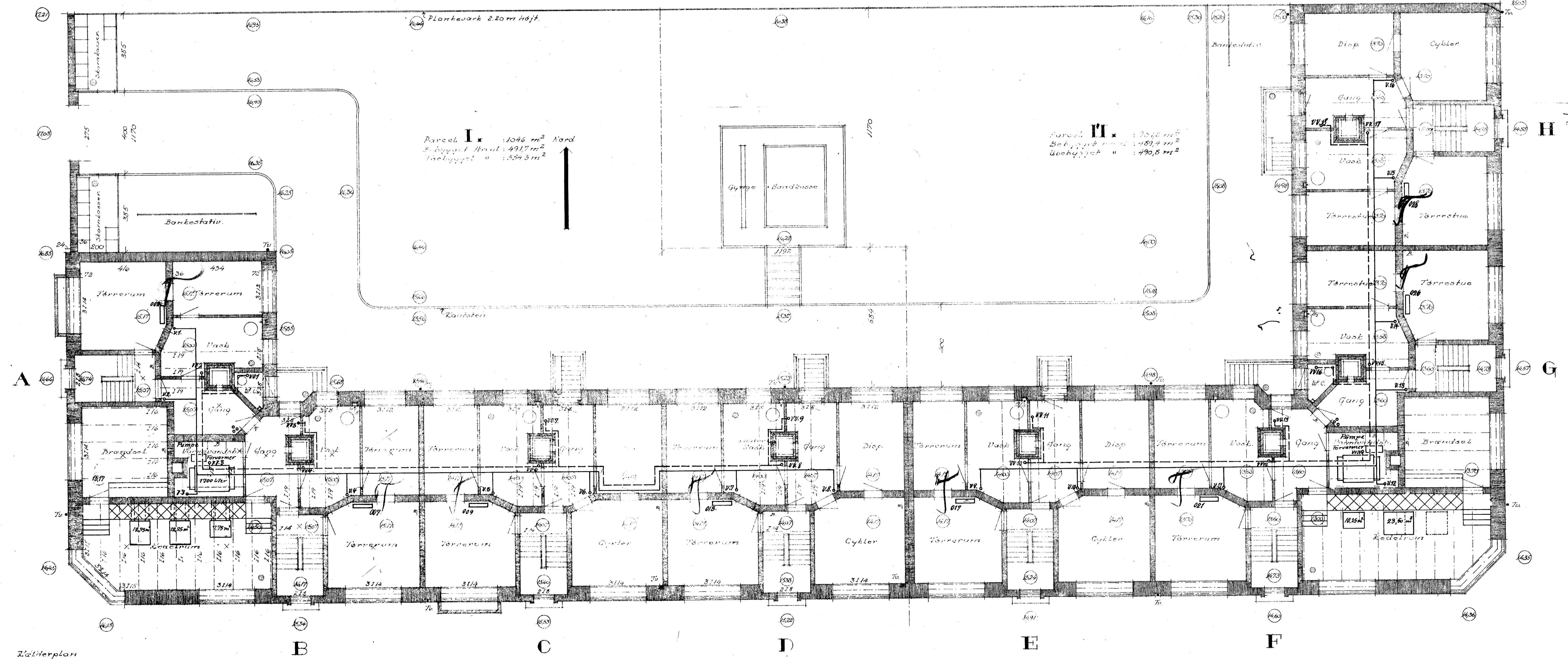
2. etageplan
